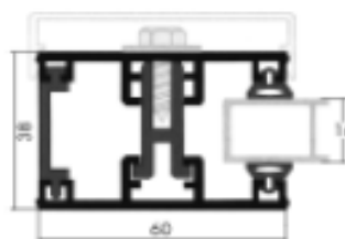
Profili ristlõige.
