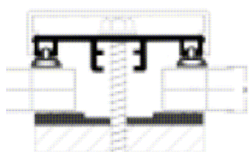
Profili ristlõige.
